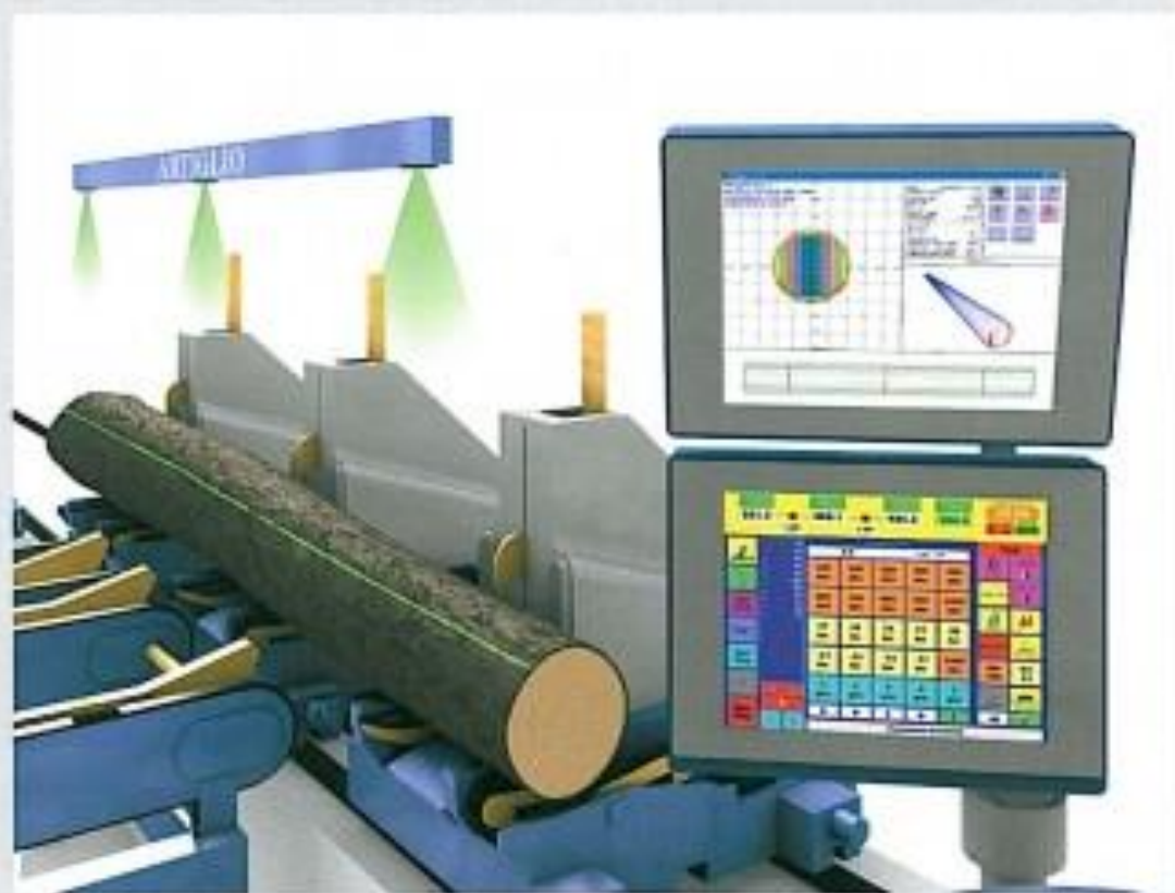
Système de vision en 3D de la grume avec calcul du volume et optimisation de coupe
